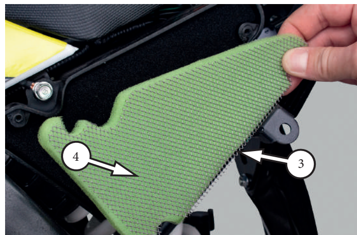
Фото 5.7. Обслуживание воздушного фильтра закрытого типа
