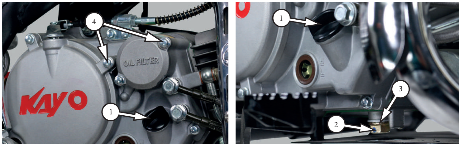
Фото 5.5. Замена моторного масла в двигателях с масляным фильтром и смотровым окном
