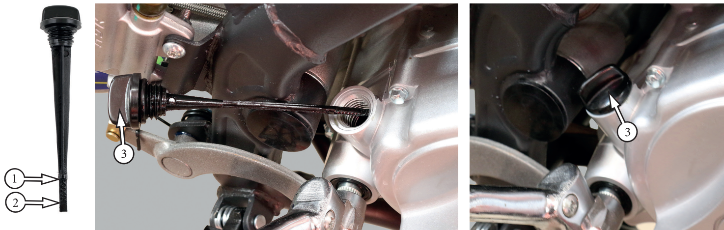
Фото 5.3. Указатель уровня масла в двигателях
