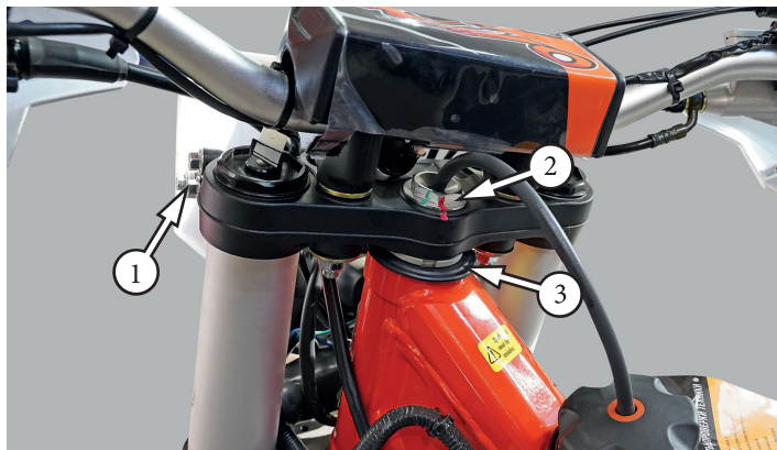
Фото 5.33. Регулировка подшипников рулевой колонки
