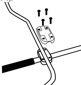
Рис. 4 Установка рукояток
