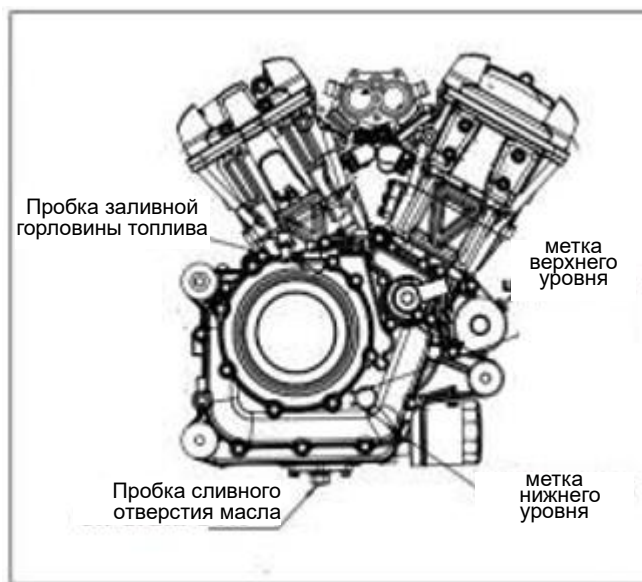
Рис. 15 Проверка уровня масла
