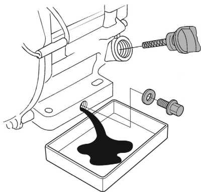
Рис. 29 Замена масла в двигателе
