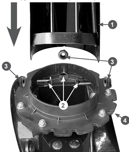
Рис. 14 Установка жёлоба выброса снега
