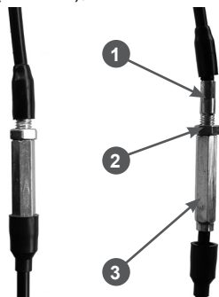
Рис. 13 Механизм регулировки тросов
