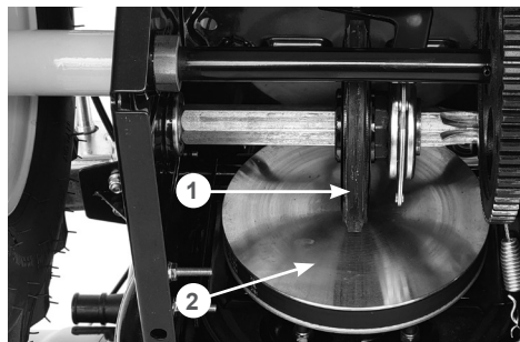
Рис. 12 Проверка нейтрального положения фрикционного колеса
