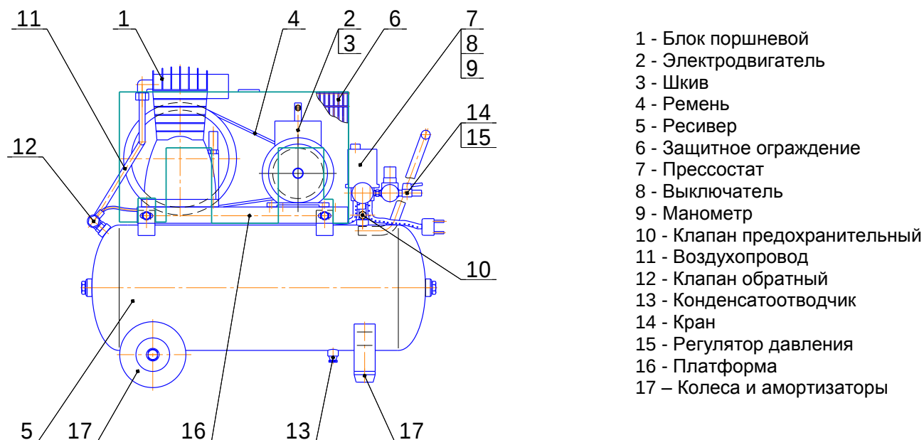
Рисунок 5 - Общий вид компрессора СБ4/С-50.LH20A-1.5, СБ4/С-50.LH20, СБ4/С-50.LH20A
