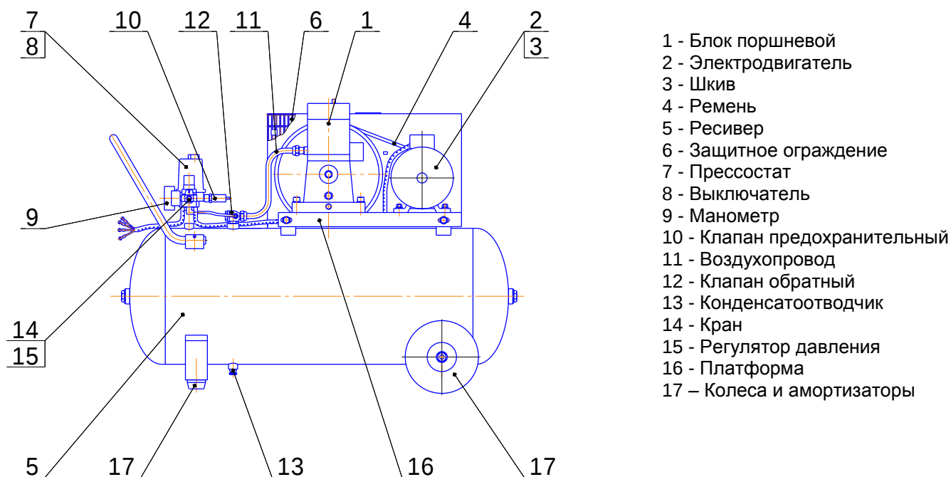
Рисунок 6 - Общий вид компрессора СБ4/С-100.LH20A-1.5, СБ4/С-100.LH20, СБ4/С-100.LH20A
