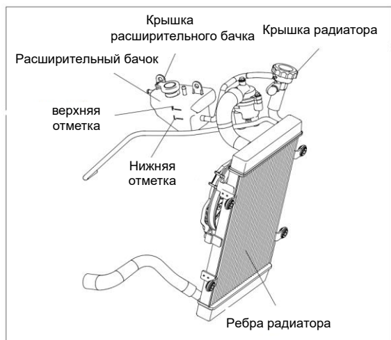
Рис. 40 Система охлаждения
