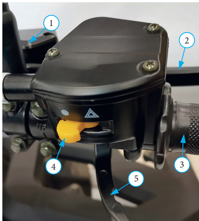
Фото 2.5.1 Переключатели правого рулевого блока квадрицикла:
