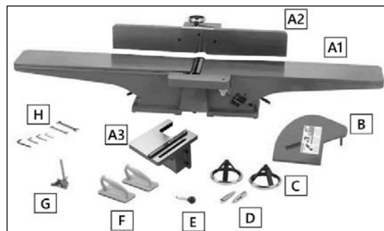
Рисунок 2. Содержимое упаковки 2
