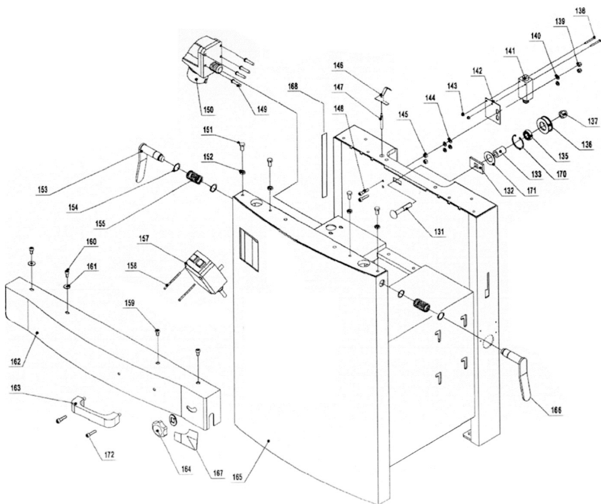
Рисунок 30. Основание станка
