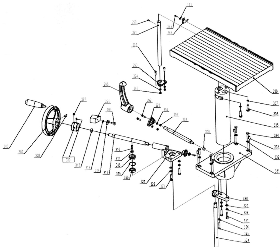
Рисунок 32. Стол рейсмусовый
