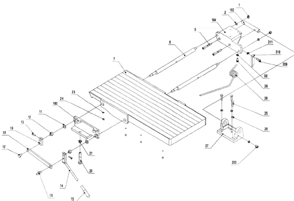
Рисунок 28. Стол загрузочный
