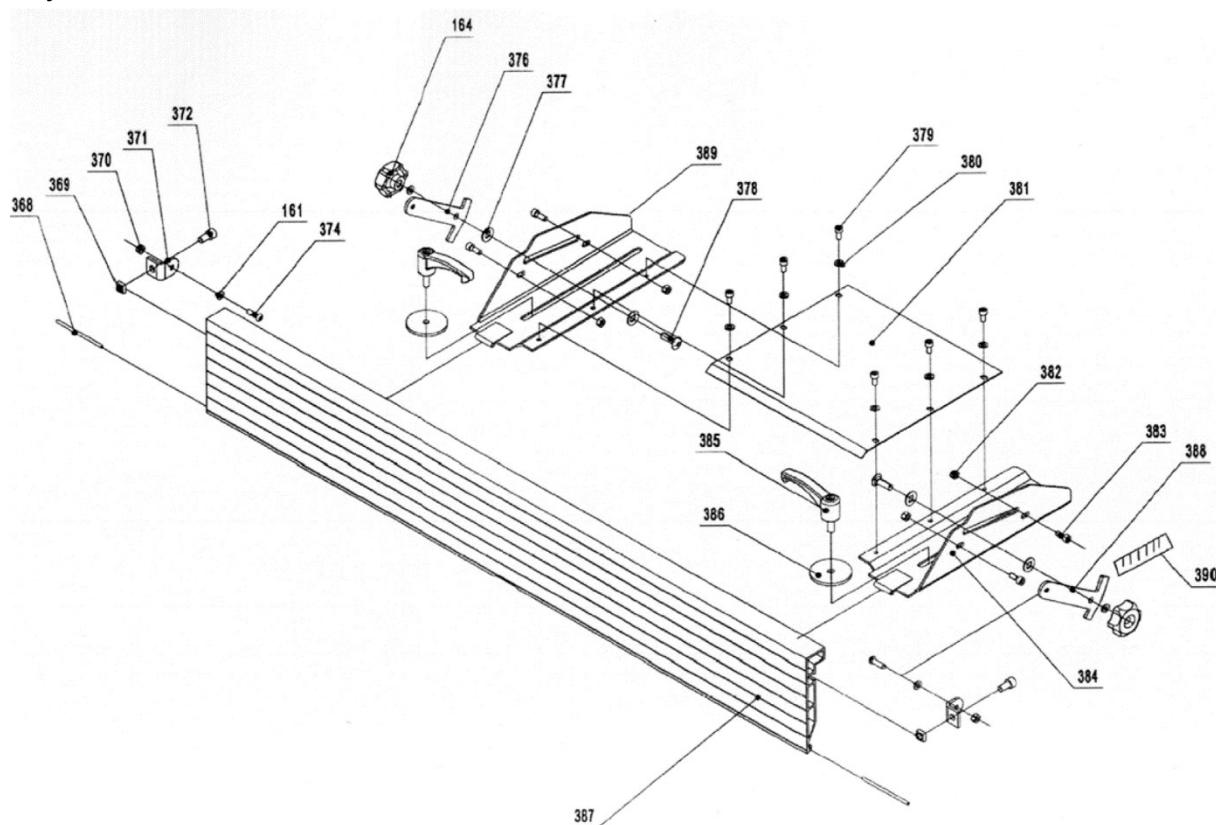
Рисунок 31. Параллельный упор
