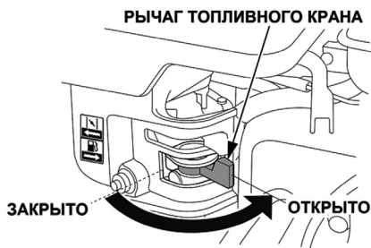
Рис. 8 Топливный кран открыт
