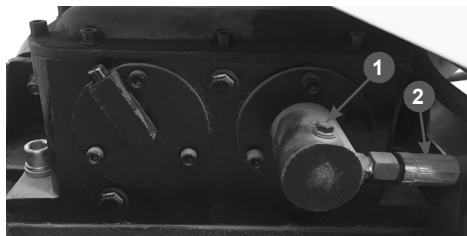
Рис. 23 Пробка для удаления воздуха из системы гидравлического привода 1. Пробка для удаления воздуха из системы гидравлического привода 2. Шланг системы гидравлического привода
