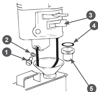
Рис. 18 Обслуживание фильтра-отстойника
