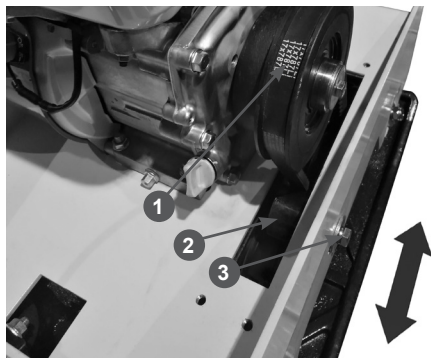
Рис. 25 Регулировка натяжения ремня
