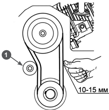
Рис. 24 Проверка натяжения ремня привода вибратора 1. Ролик натяжения ремня
